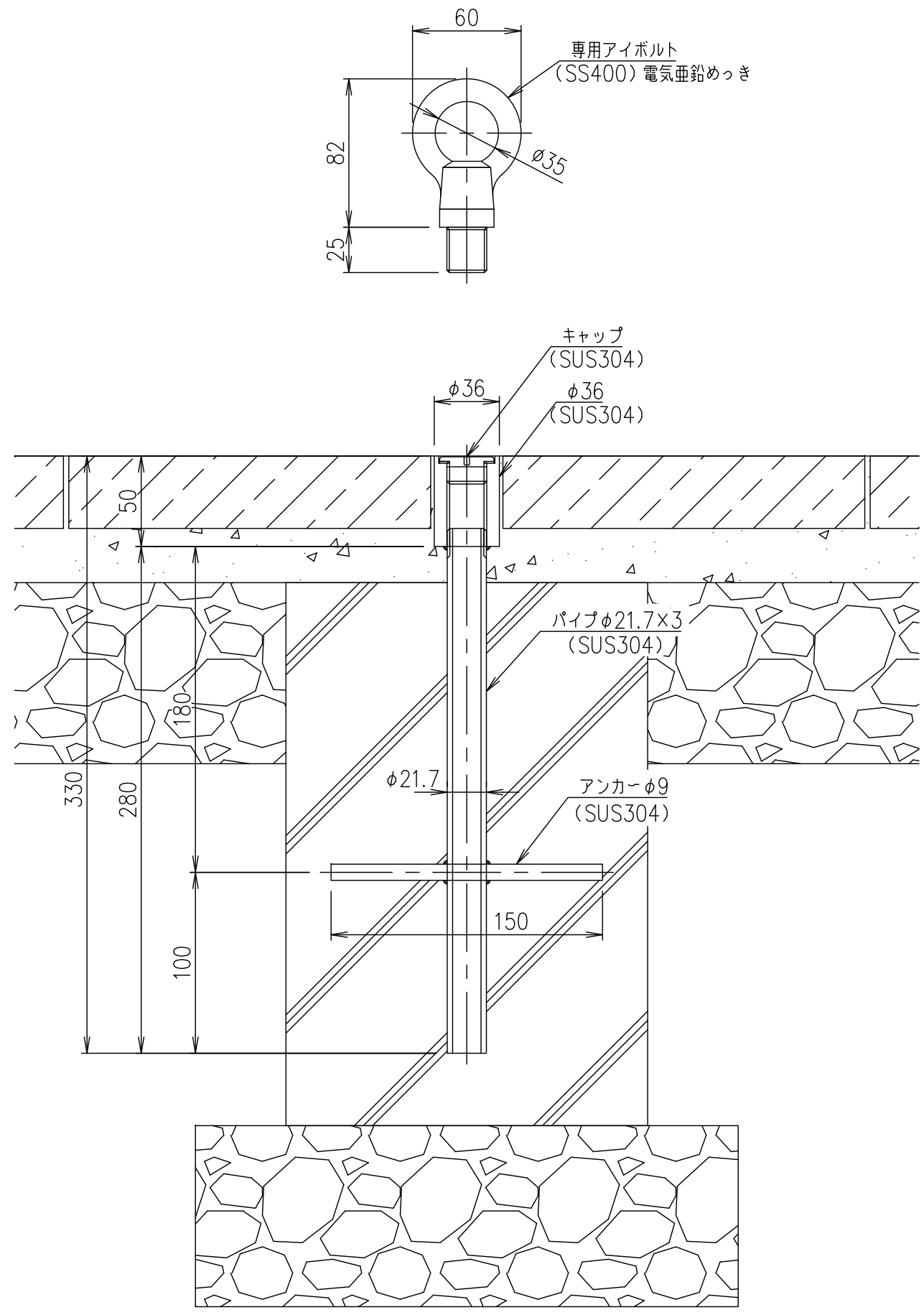
施工図 (参考)
