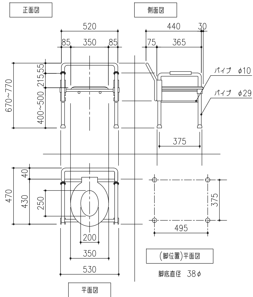
使用状態寸法図 (参考図)
