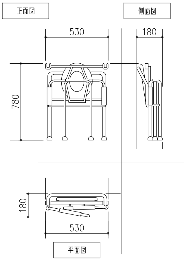
収納時寸法図 (参考図)
