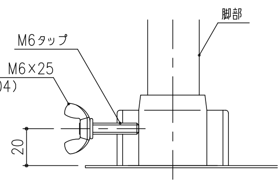
A部拡大詳細図 S=1/2
