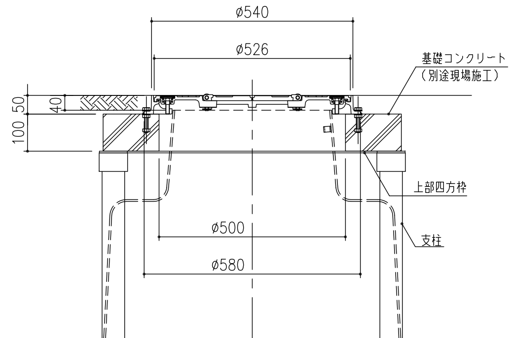
施工断面図
