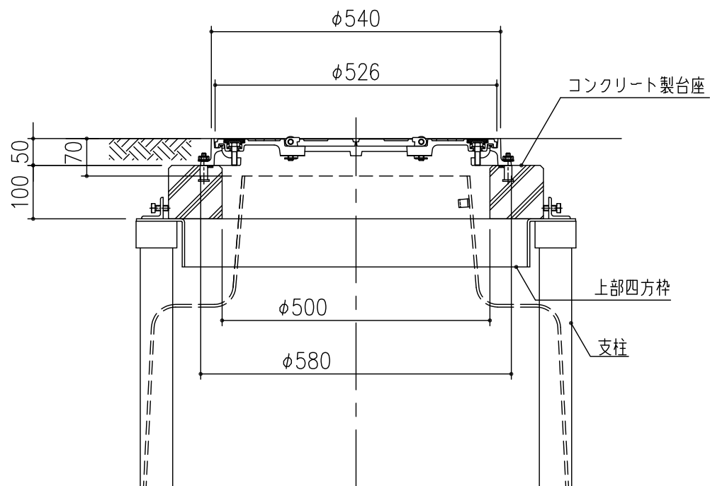
施工断面図
