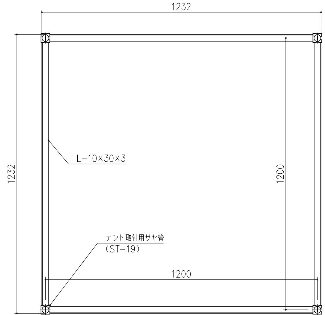
製品平面図 S=1/10
