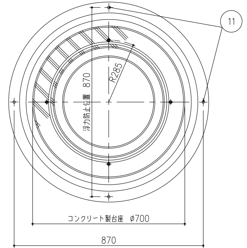
平面図(コンクリート製台座・便槽のみ)
