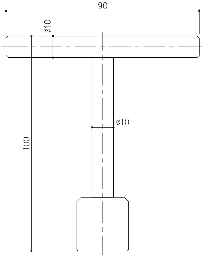
特殊ボルト専用ハンドル M10L-F
