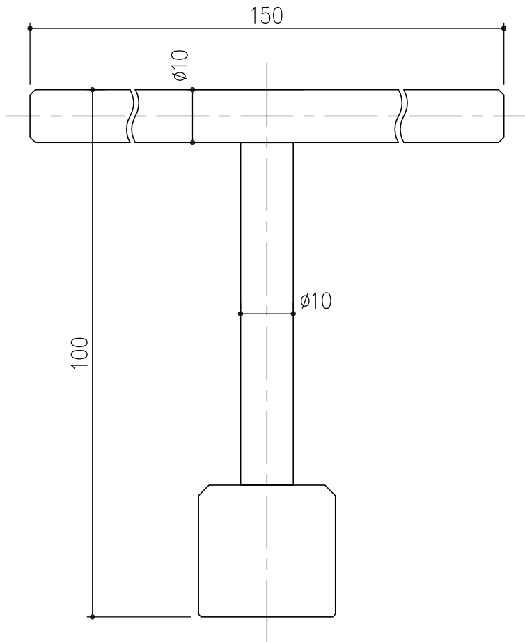
特殊ボルト専用ハンドル M12L-F
