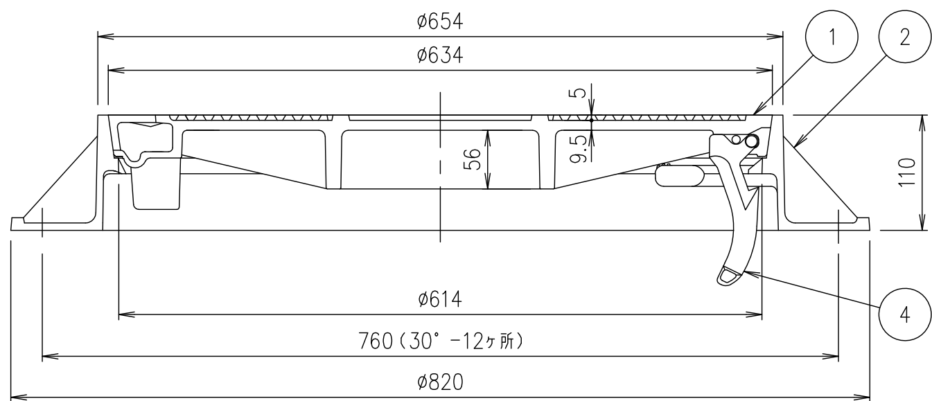
A-A断面図
