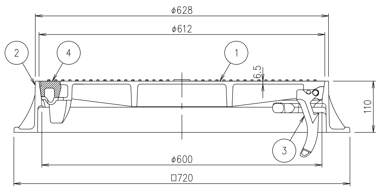
A-A断面
