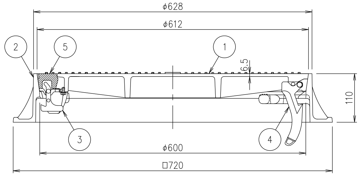
A-A断面
