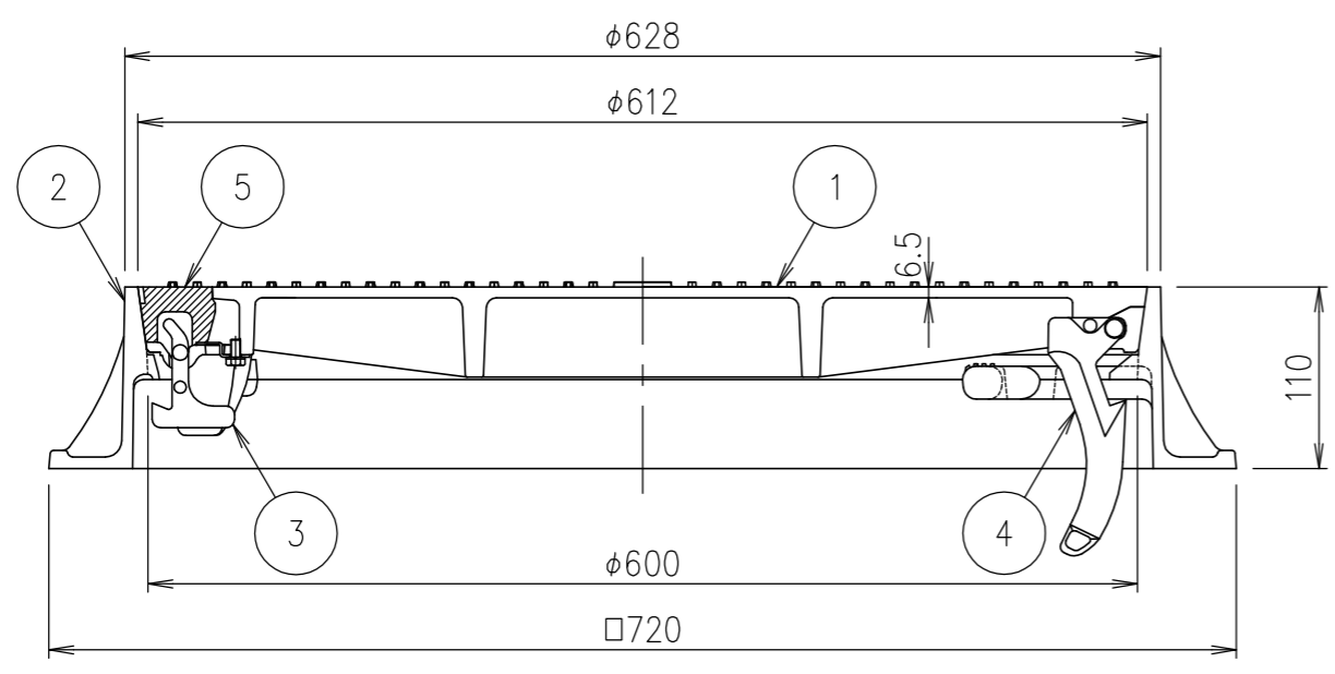
A-A断面
