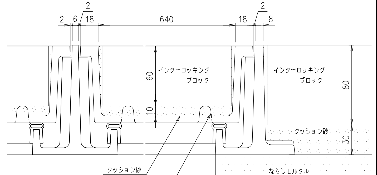
施工部分図
