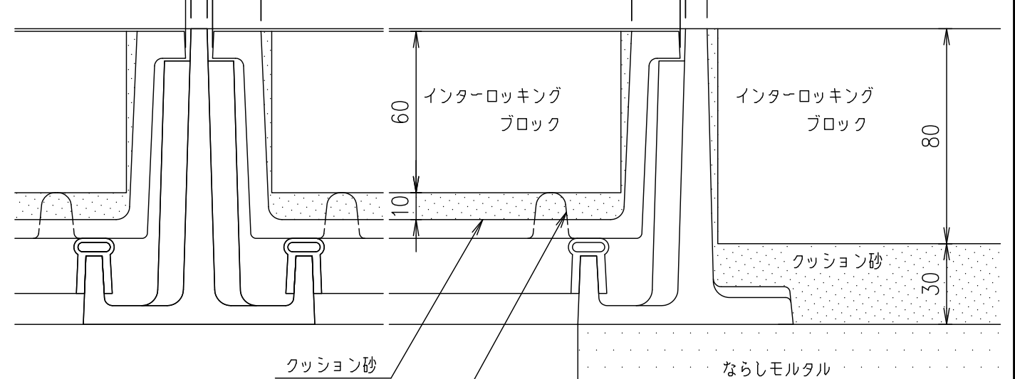
施工部分図
