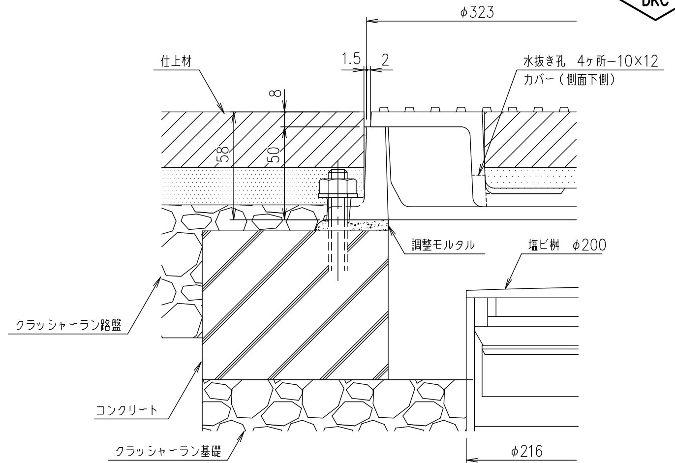
施工参考断面図 S=1/2
