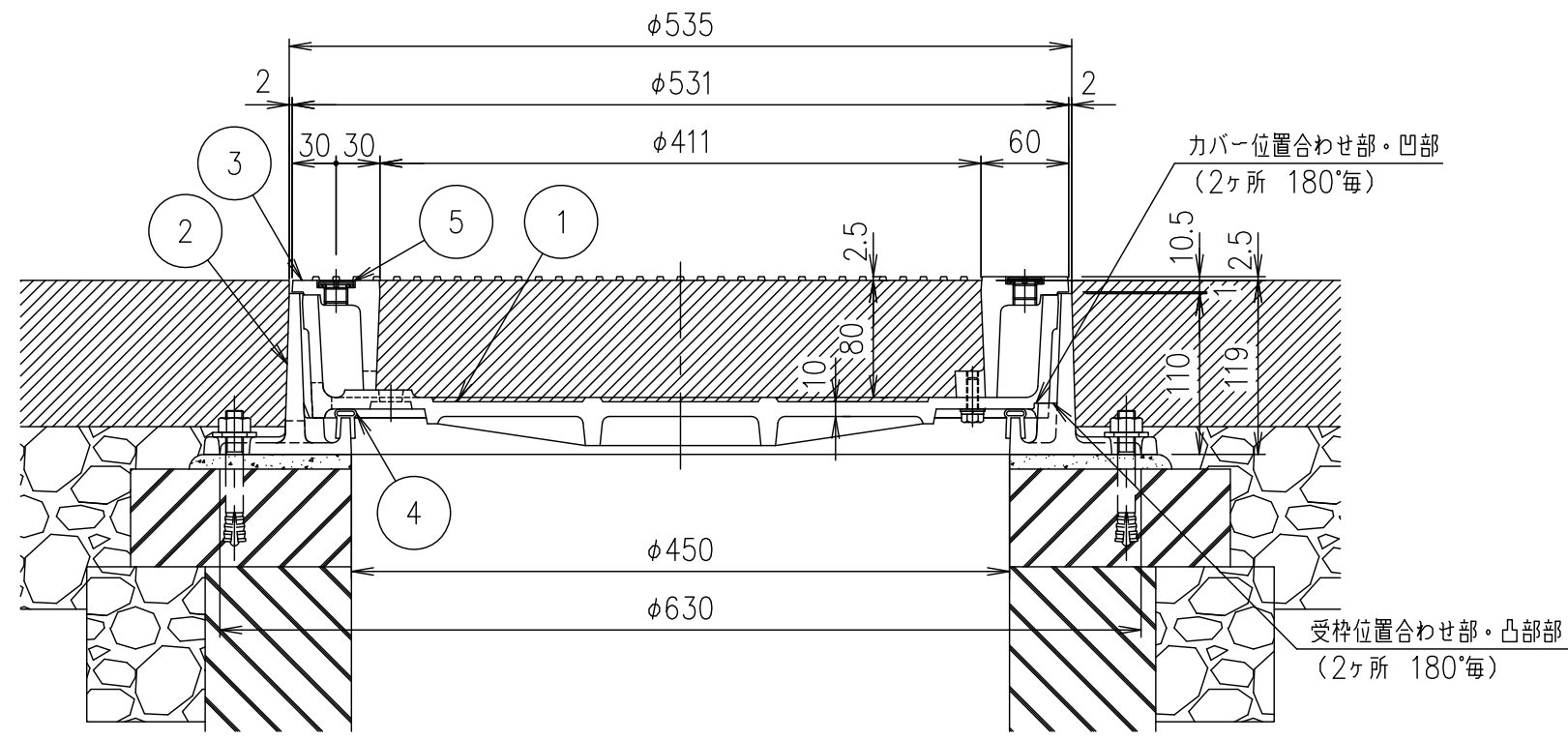
エンボス模様断面詳細 S=1/1
