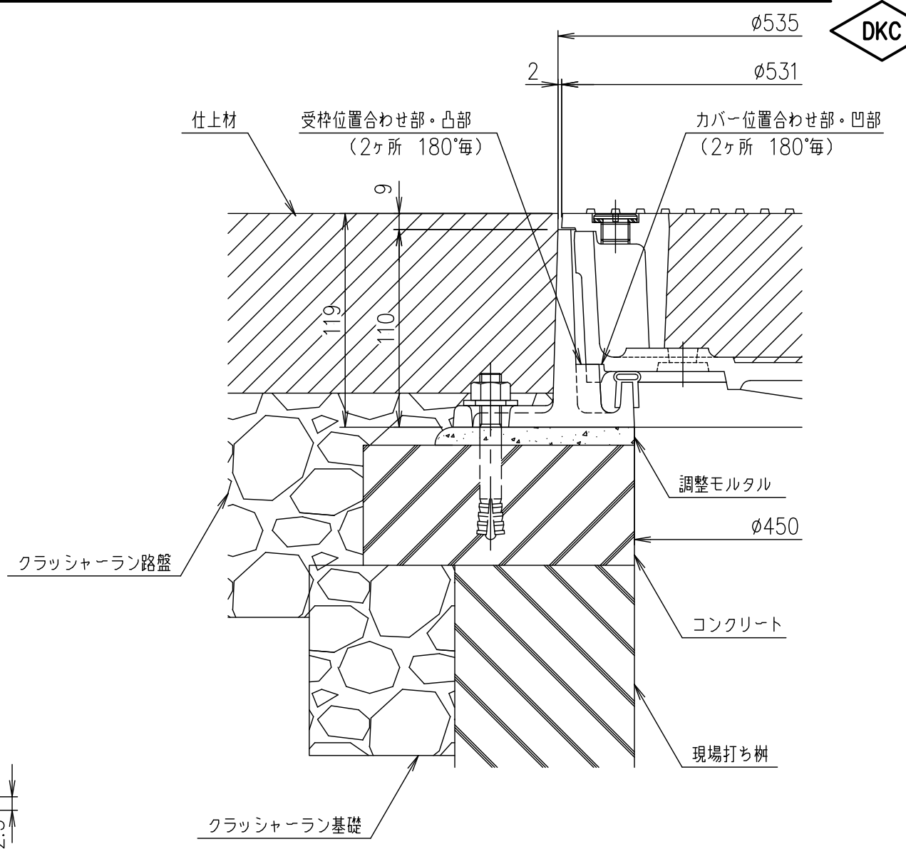
エンボス模様断面詳細 S=1/1
