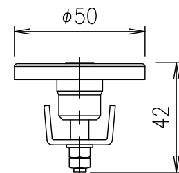
ロック錠断面図 S=1/2
