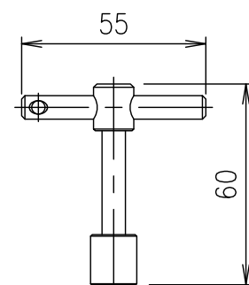
ロック錠専用鍵 S=1/2 MF-43
