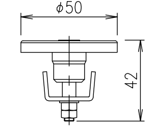
ロック錠断面図 S=1/2 LO-F
