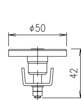
ロック錠断面図 S=1/2 LO-F
