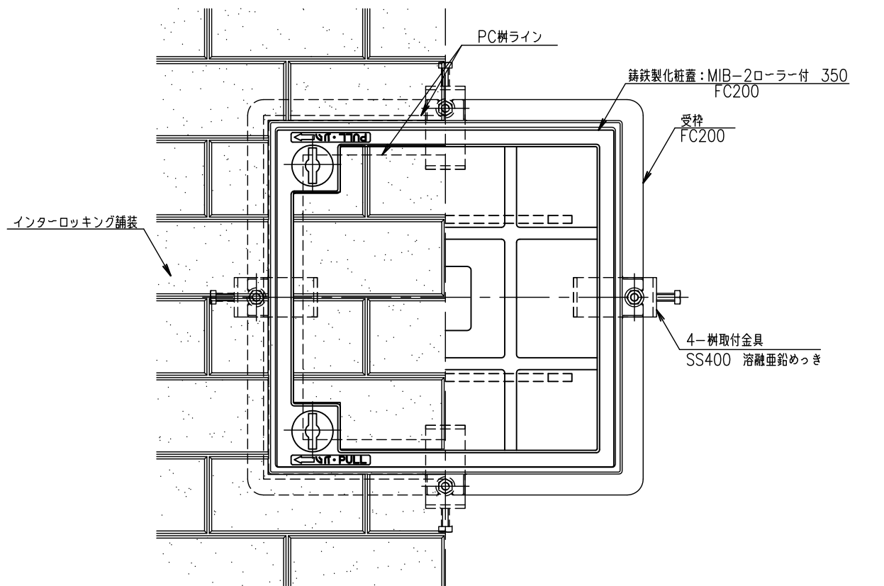
平面図
