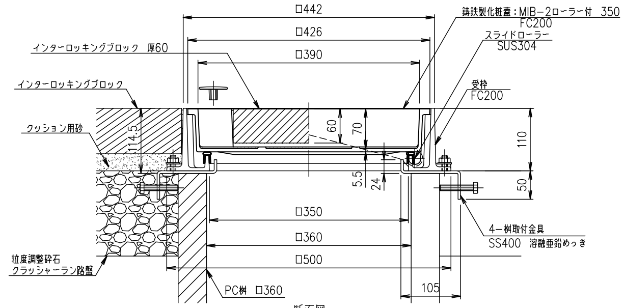
断面図
