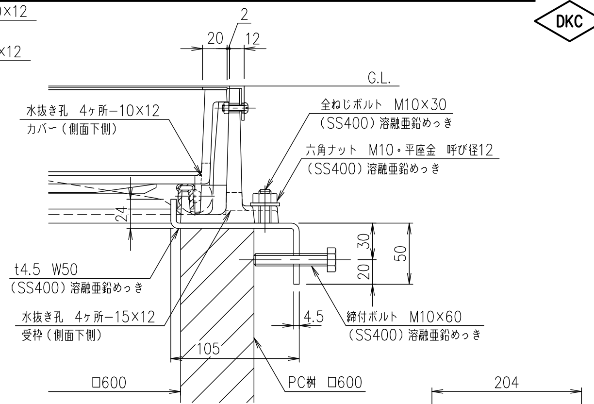
柵取付金具詳細図 S=1/3
