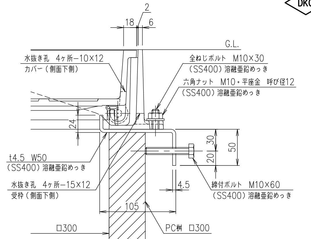
桷取付金具詳細図 S=1/3
