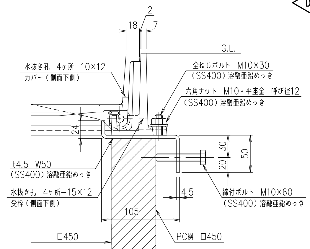
桷取付金具詳細図 S=1/3
