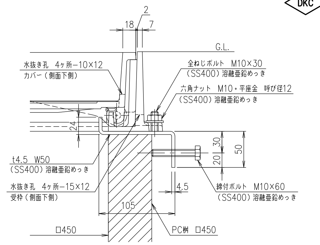
樹取付金具詳細図 S=1/3
