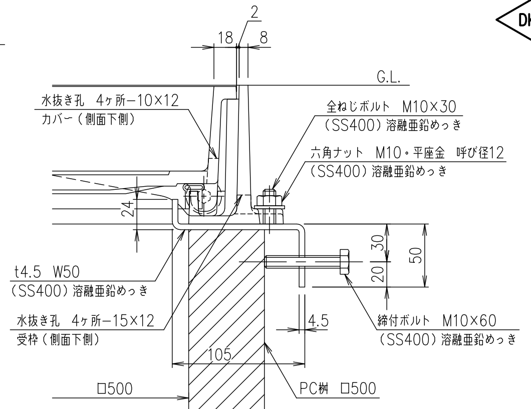
樹取付金具詳細図 S=1/3
