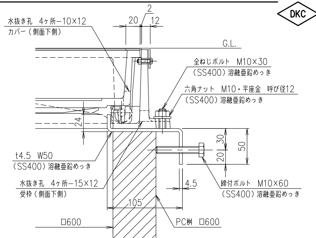
柵取付金具詳細図 S=1/3
