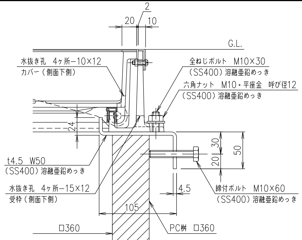
枡取付金具詳細図 S=1/3
