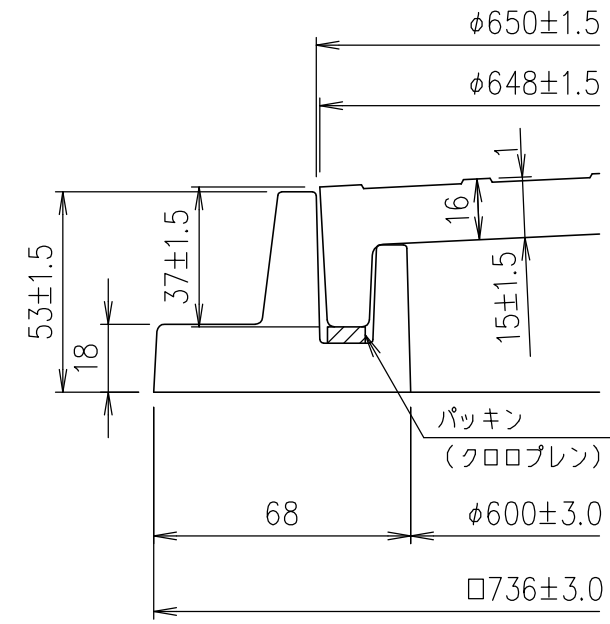
蓋・受枠断面詳細図
