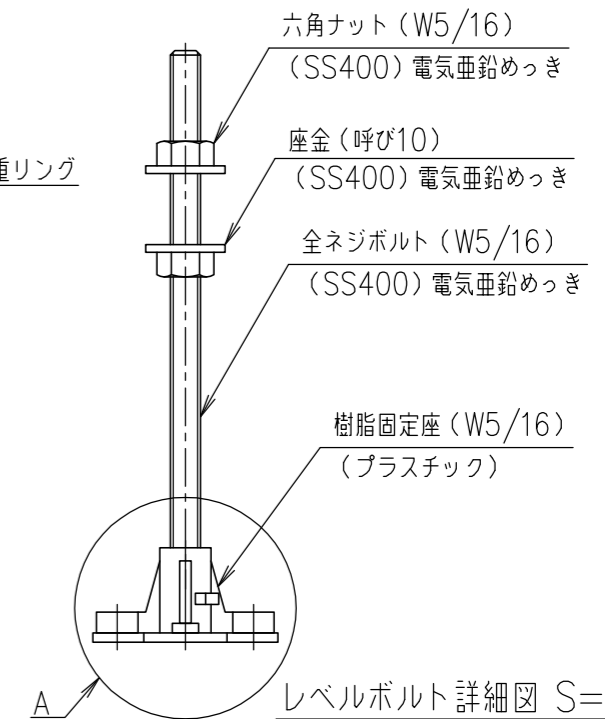
A部詳細図 S=1/2
