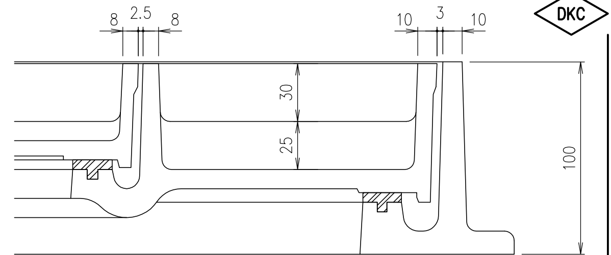
部分詳細図 S=1/2
