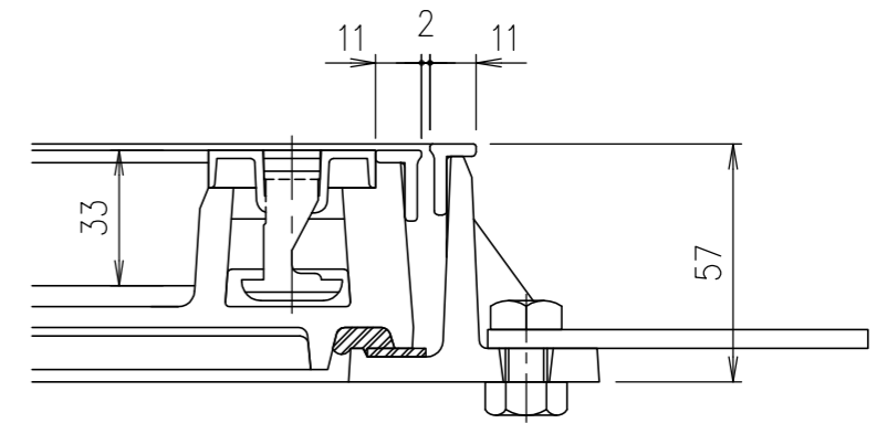
部分詳細図 S=1/2
