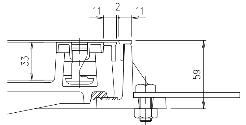
部分詳細図 S=1/2
