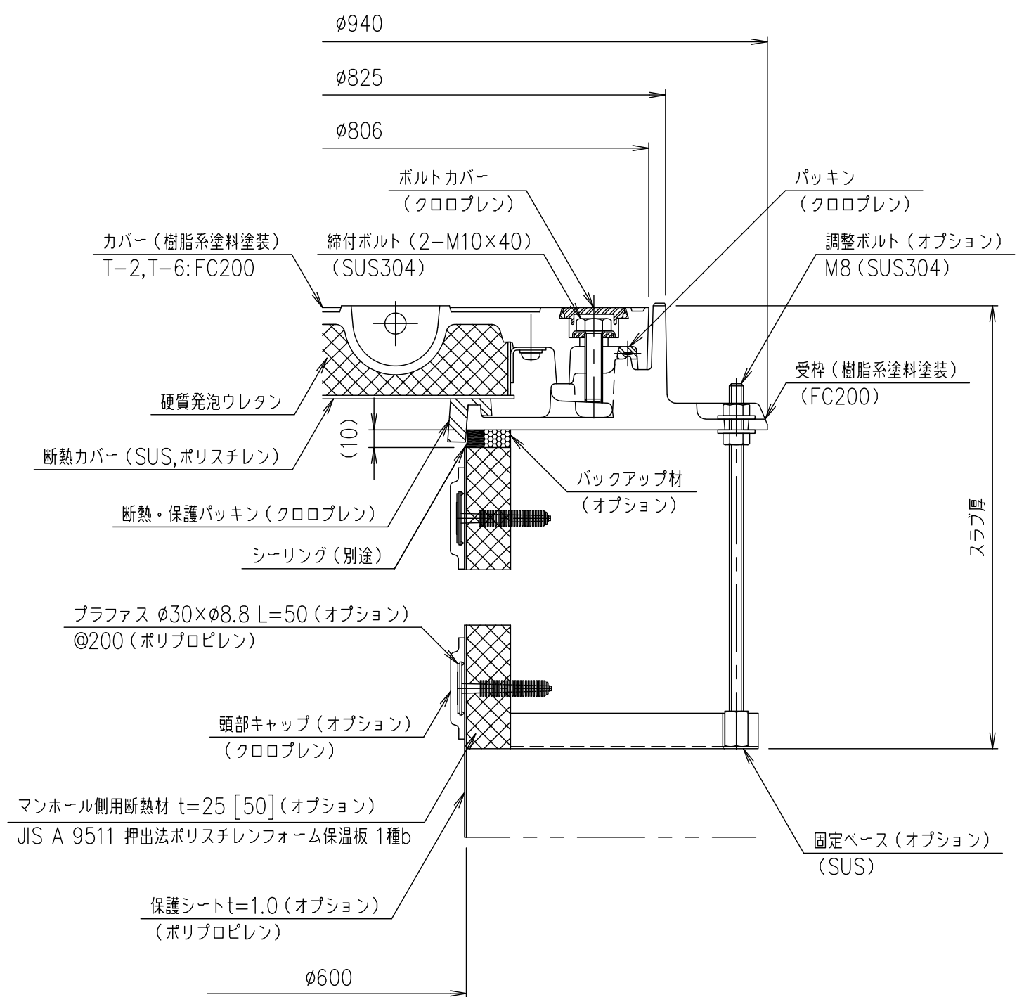
B-B断面図 S=1/3
