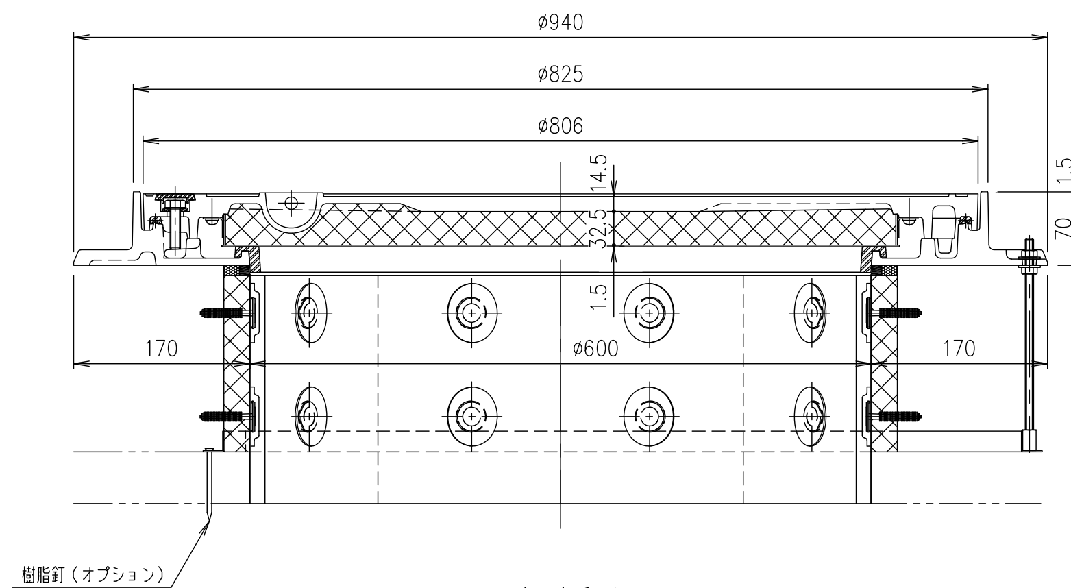
A-A断面図
