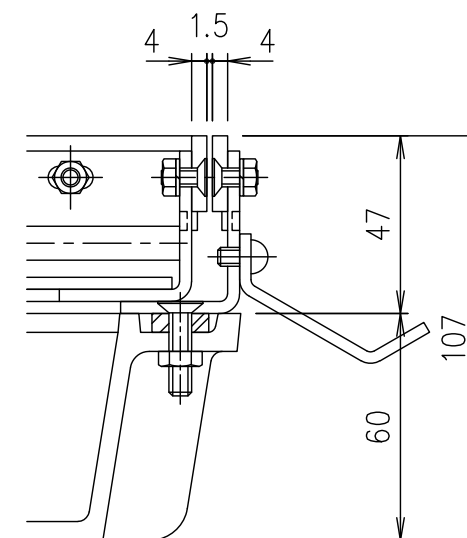
部分詳細図 S=1/2
