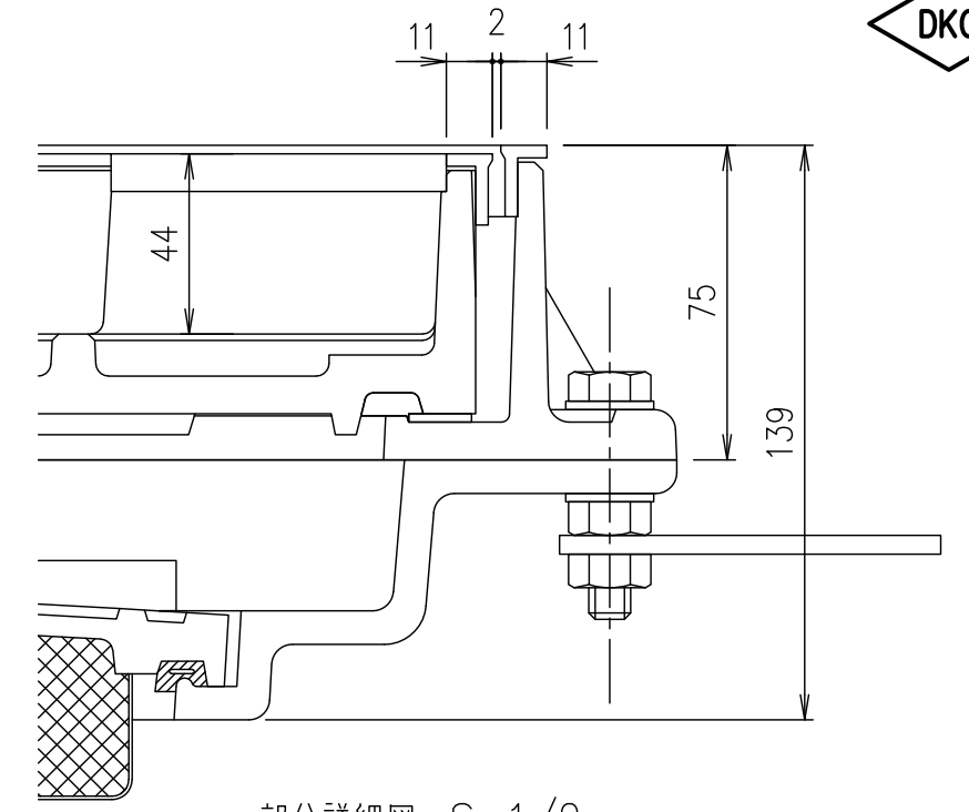
部分詳細図 S=1/2
