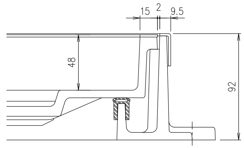
部分詳細図 S=1/2
