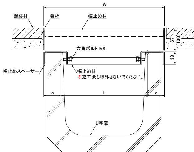
納まり例
