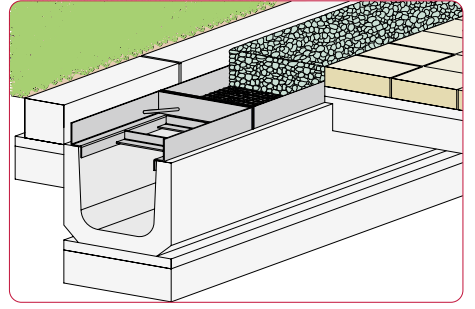
●植栽地—緑石—側溝—舗装
