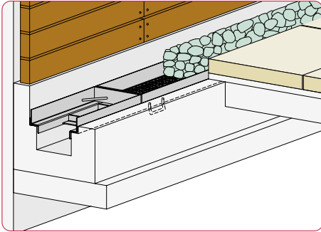
●建物—側溝—舗装
