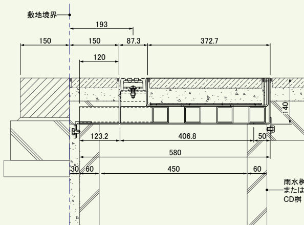
溝内偏芯バウンダリー樹用 T-2用・T-14(R5)用
