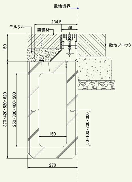
ぴったん溝(ぴったんこう) T-2用・T-25用
