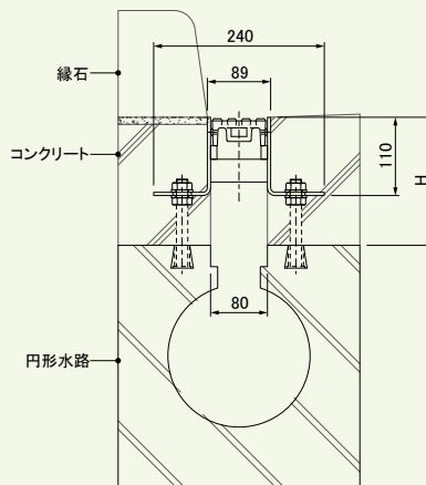
円形水路用(レベル調整タイプ) T-2用・T-14(R5)用
