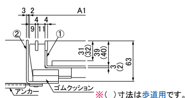
共通断面図
