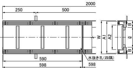
●LPSL10 寸法表
