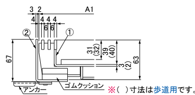
●共通断面図
