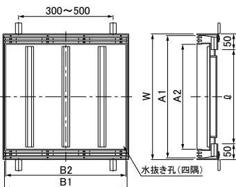
●LPSLM10 寸法表
