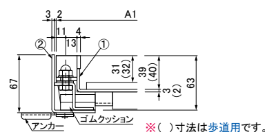
共通断面図
