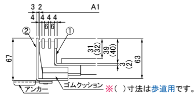
●共通断面図
