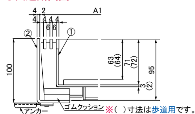
●共通断面図
