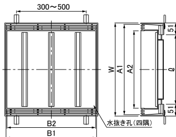
●LPSLM10H7 寸法表
