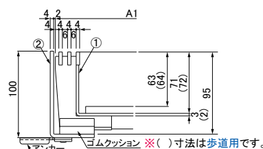
●共通断面図
