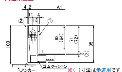
●共通断面図
