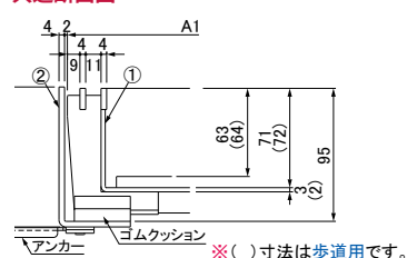
●共通断面図
