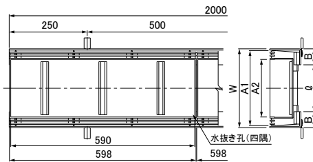
●LPSL10H7 寸法表
