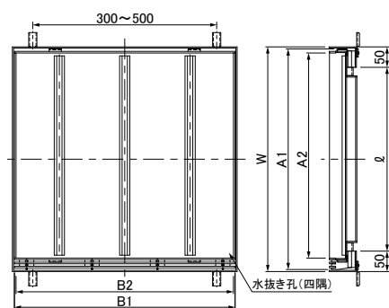
●LPSLM10片目地 寸法表
