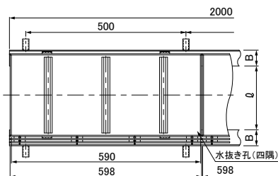
●LPSL10片目地 寸法表
