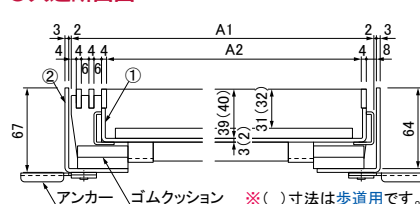
●共通断面図
