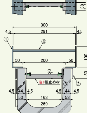
GL-100-U24 ●質量:11.6kg/m組
