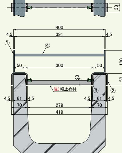
GL-100-U30 ●質量:11.7kg/m組
