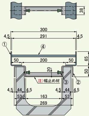
GL-65-U24 ●質量:9.1kg/m組
