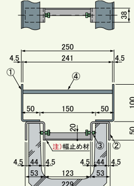
GL-100-U18 ●質量:11.5kg/m組
