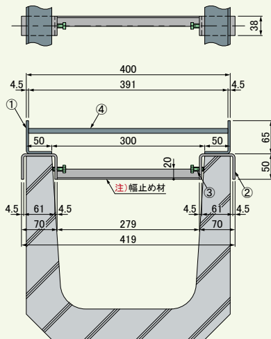
GL-65-U30 ●質量:9.2kg/m組
