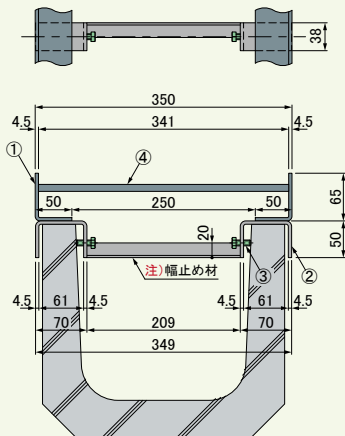
GL-65-U30 ●質量:9.2kg/m組
