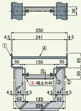
GL-65-U18 ●質量:9.0kg/m組
