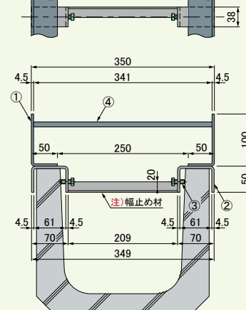
GL-100-U30 ●質量:11.7kg/m組
