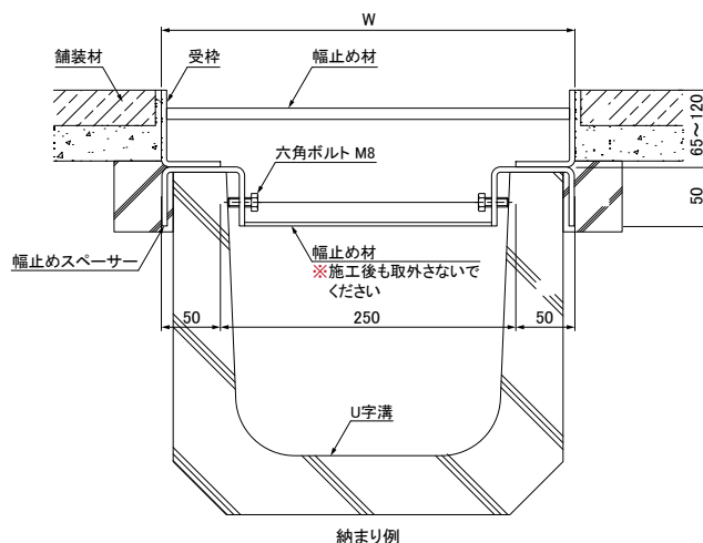
納まり例
