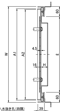
●断面図
