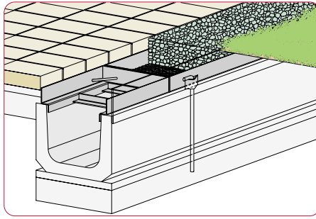
●舗装—側溝—スチールエッジ—植栽地
