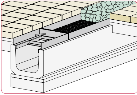
●舗装—側溝—舗装
