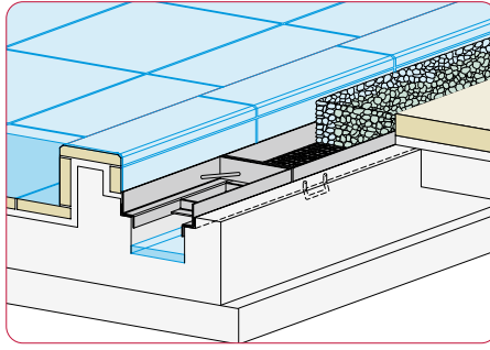
●水景—側溝—舗装
