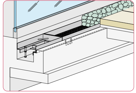
●建物—脚付き側溝—舗装
