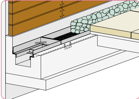
●建物—側溝—舗装
