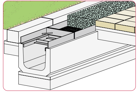
●植栽地—縁石—側溝—舗装
