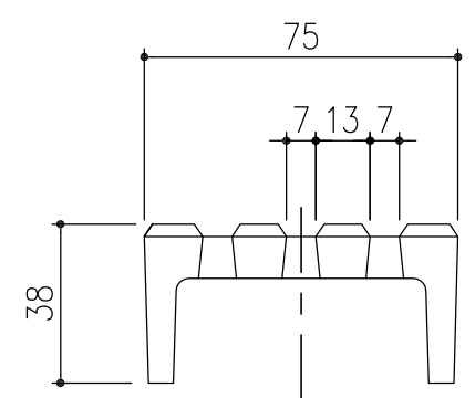
スレンダー側溝蓋 詳細図 S=1/2
