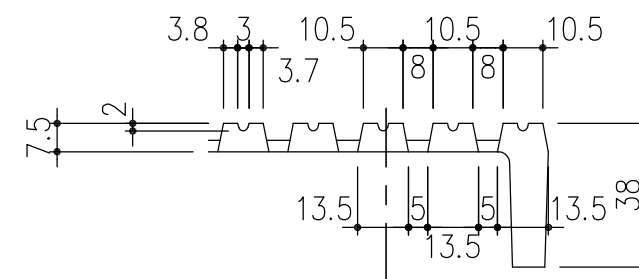
ノンスリップ詳細図 S=1/2
