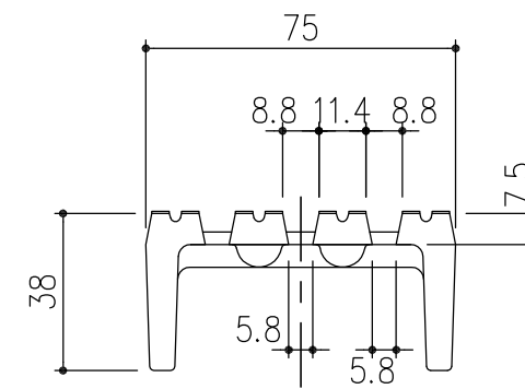
ノンスリップ詳細図 S=1/2
